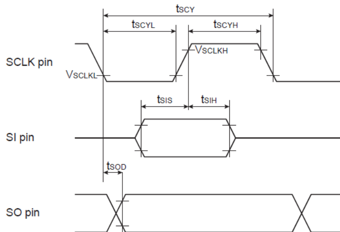
图 16.16 AC 特性图
