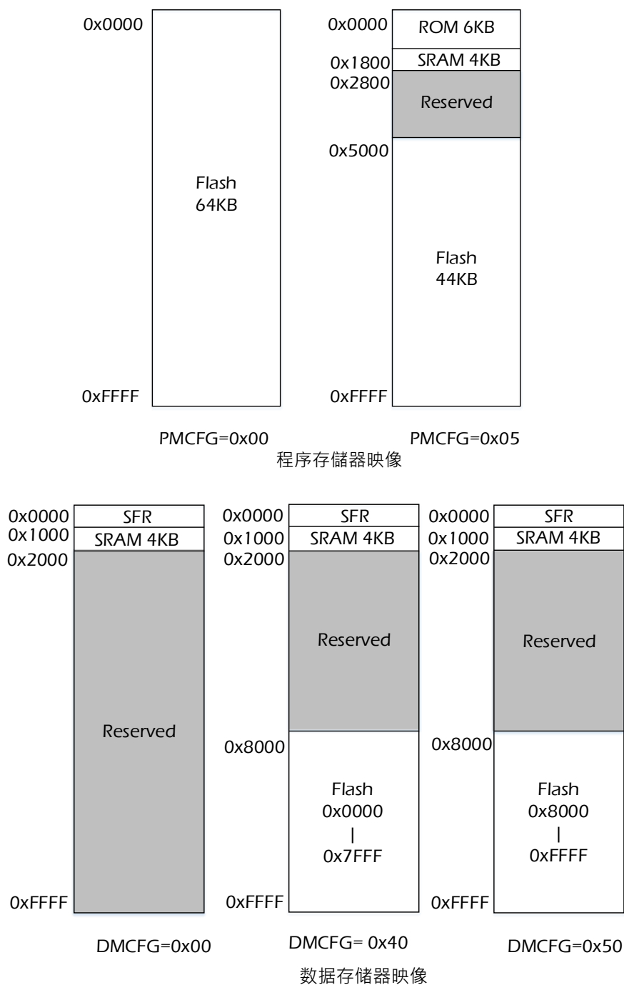
图 5.1 程序及数据存储器映像
