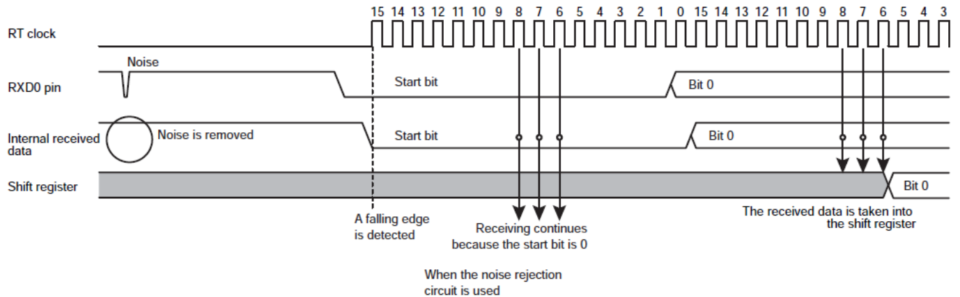
图 14.9 接收数据的噪声抑止
