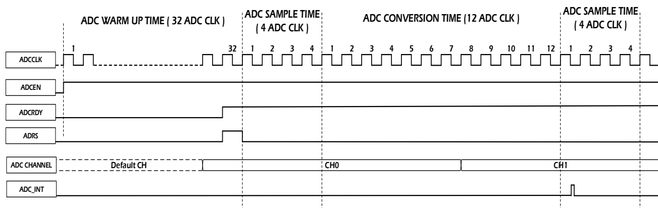
圖 8.2 ADC 上電與轉換時序圖
