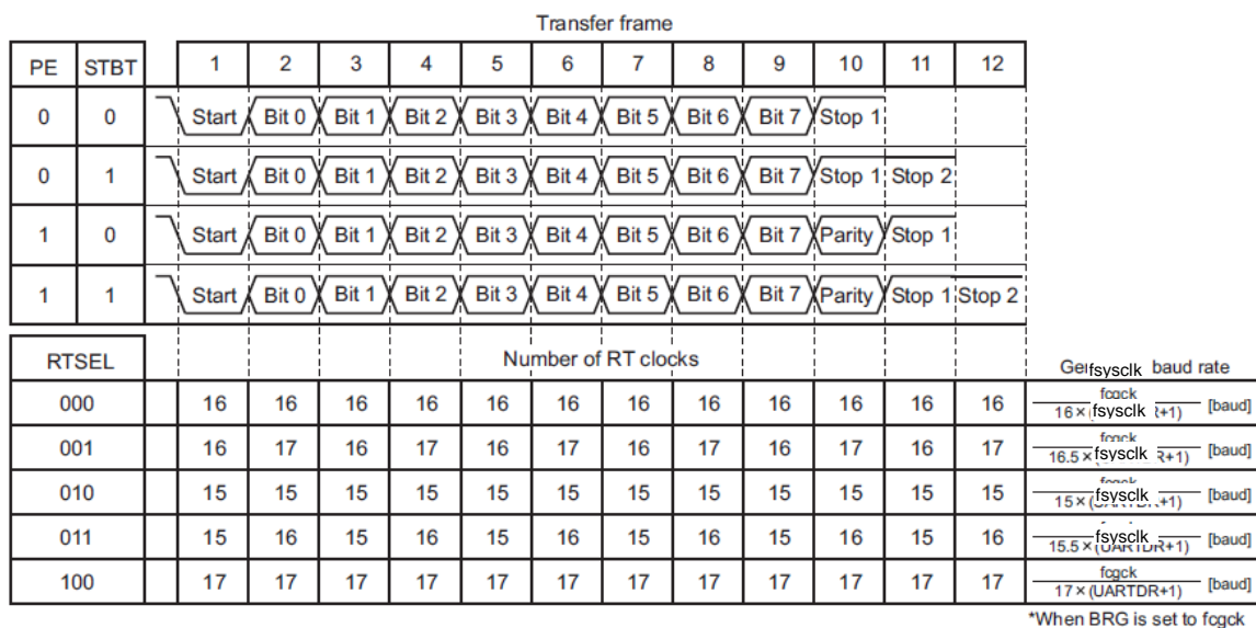
图 14.4 以 UARTxCR2<RTSEL>微调波特率
