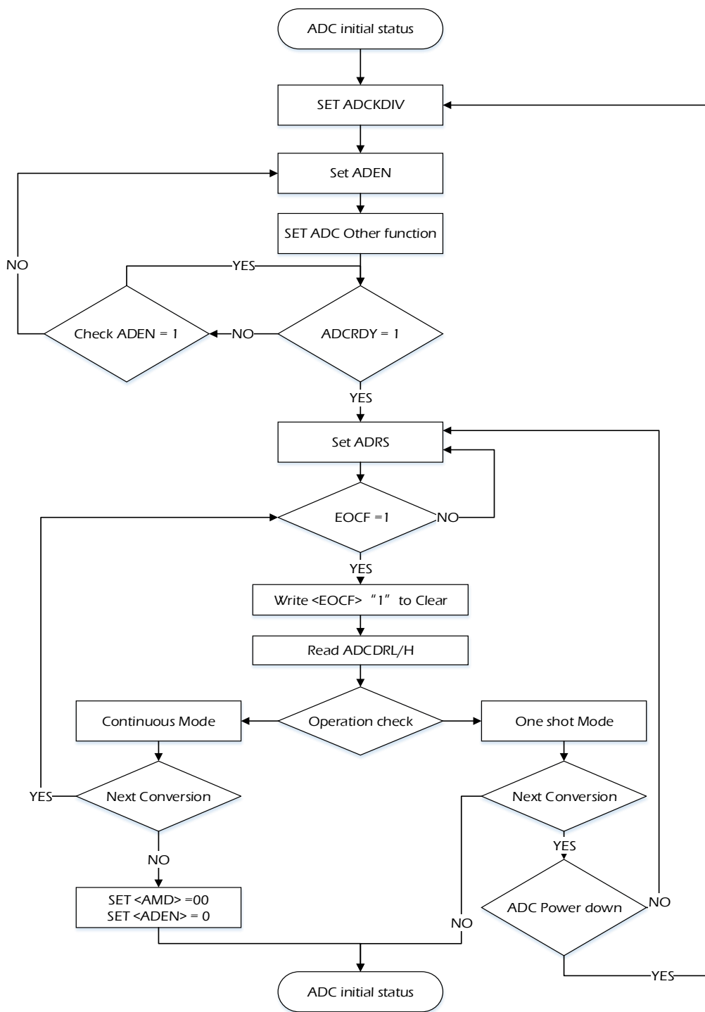
图 8.6 ADC 工作流程示意图
