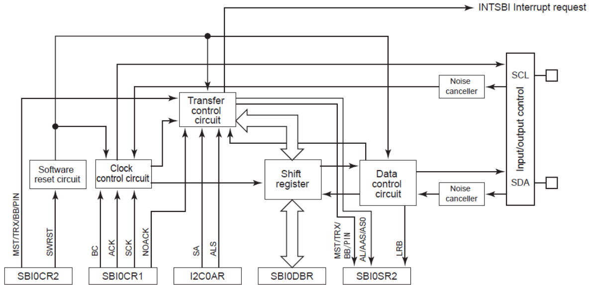
图 15.4 串行总线接口 0 (SBI0)方框图
