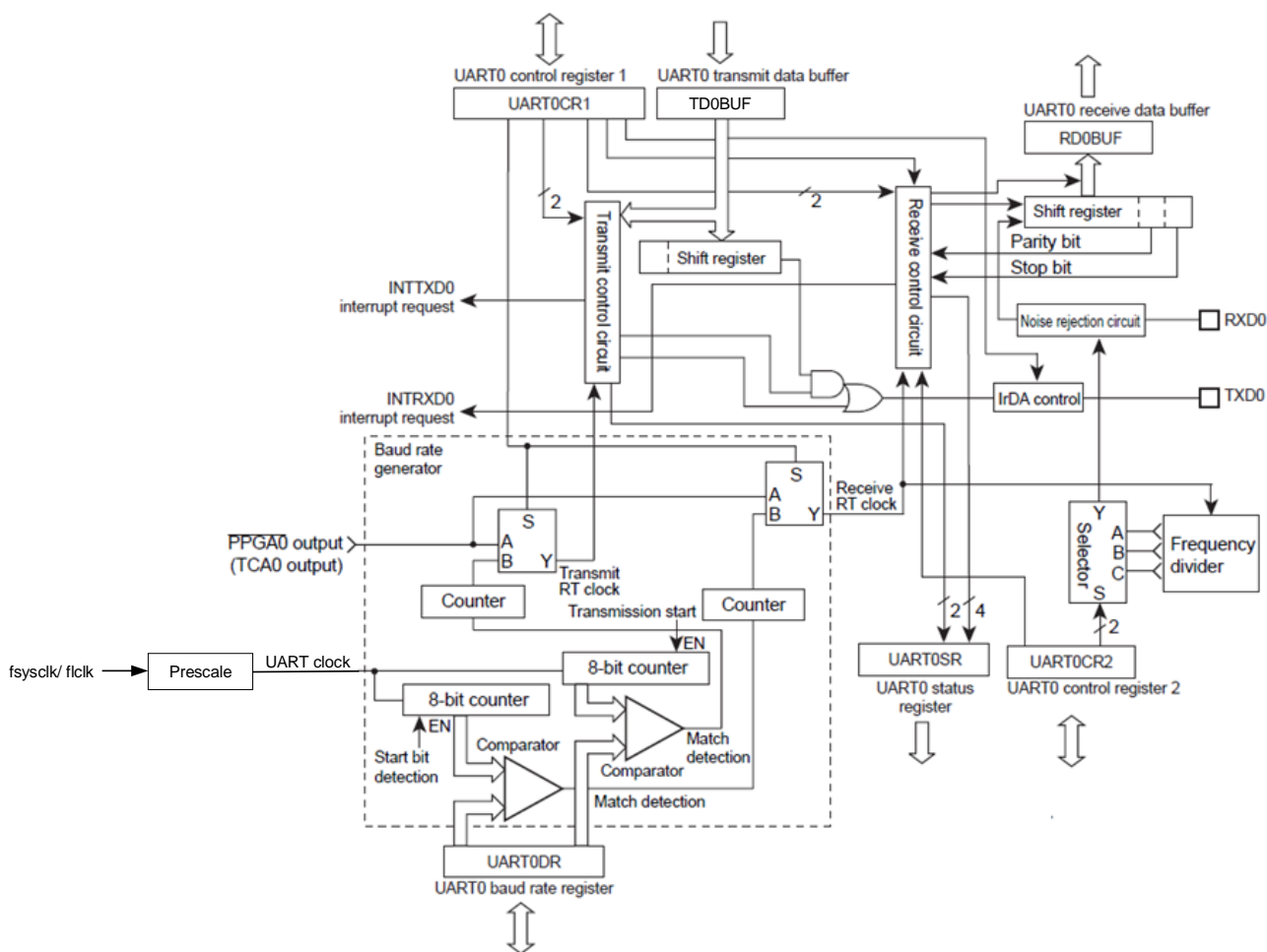
图 14.1 UART 工作模块图
