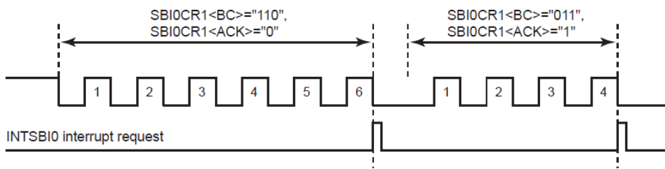
图 15.5 数据传输时的时钟脉冲与 SBIXCR1<BC>, SBIXCR1<ACK>(图以 SBIO 作为范例)
