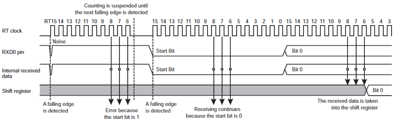
图 14.8 起始位的取样
