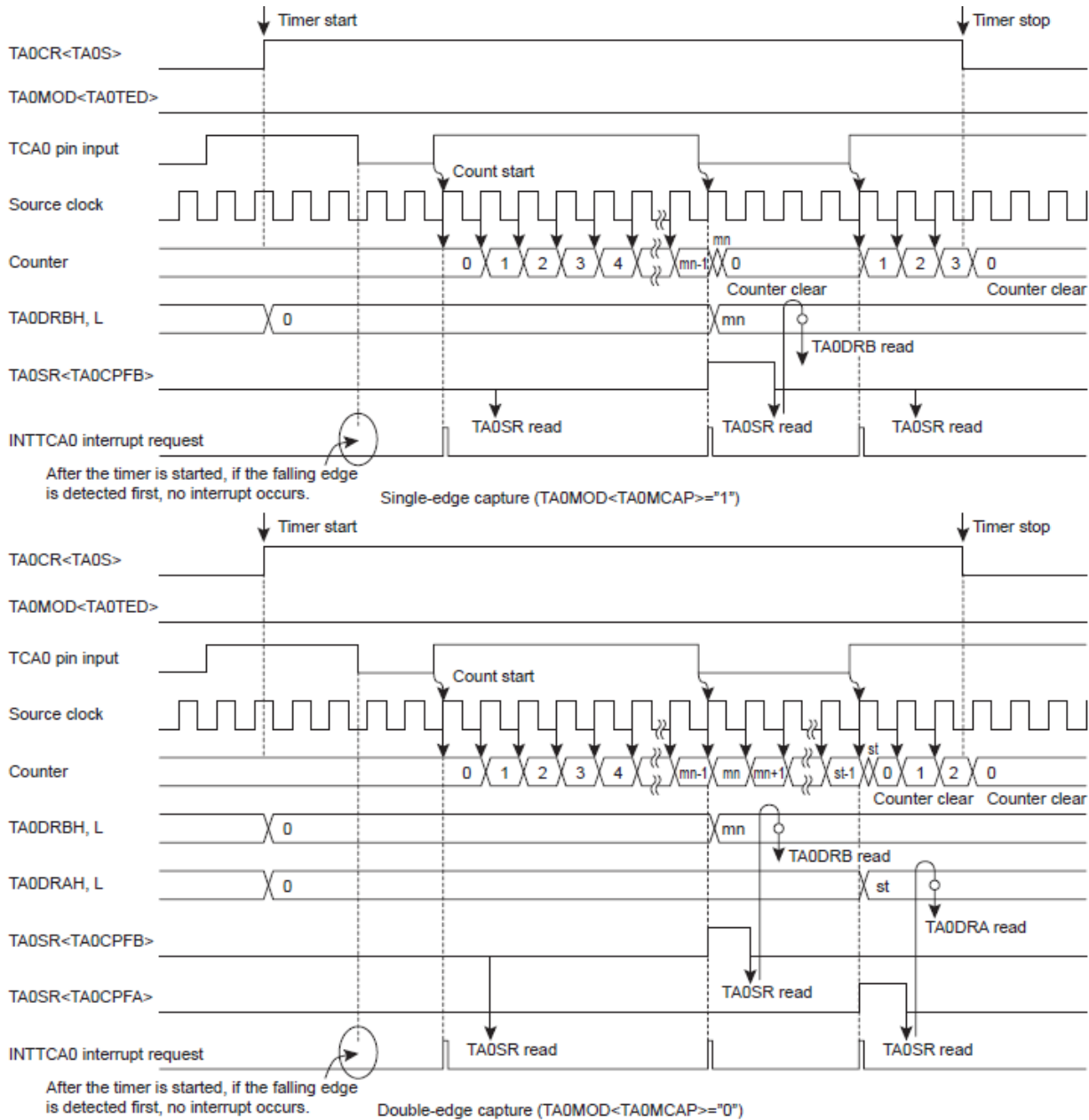
图 13.19 脉宽测量模式时序图(TCA0 为范例)
