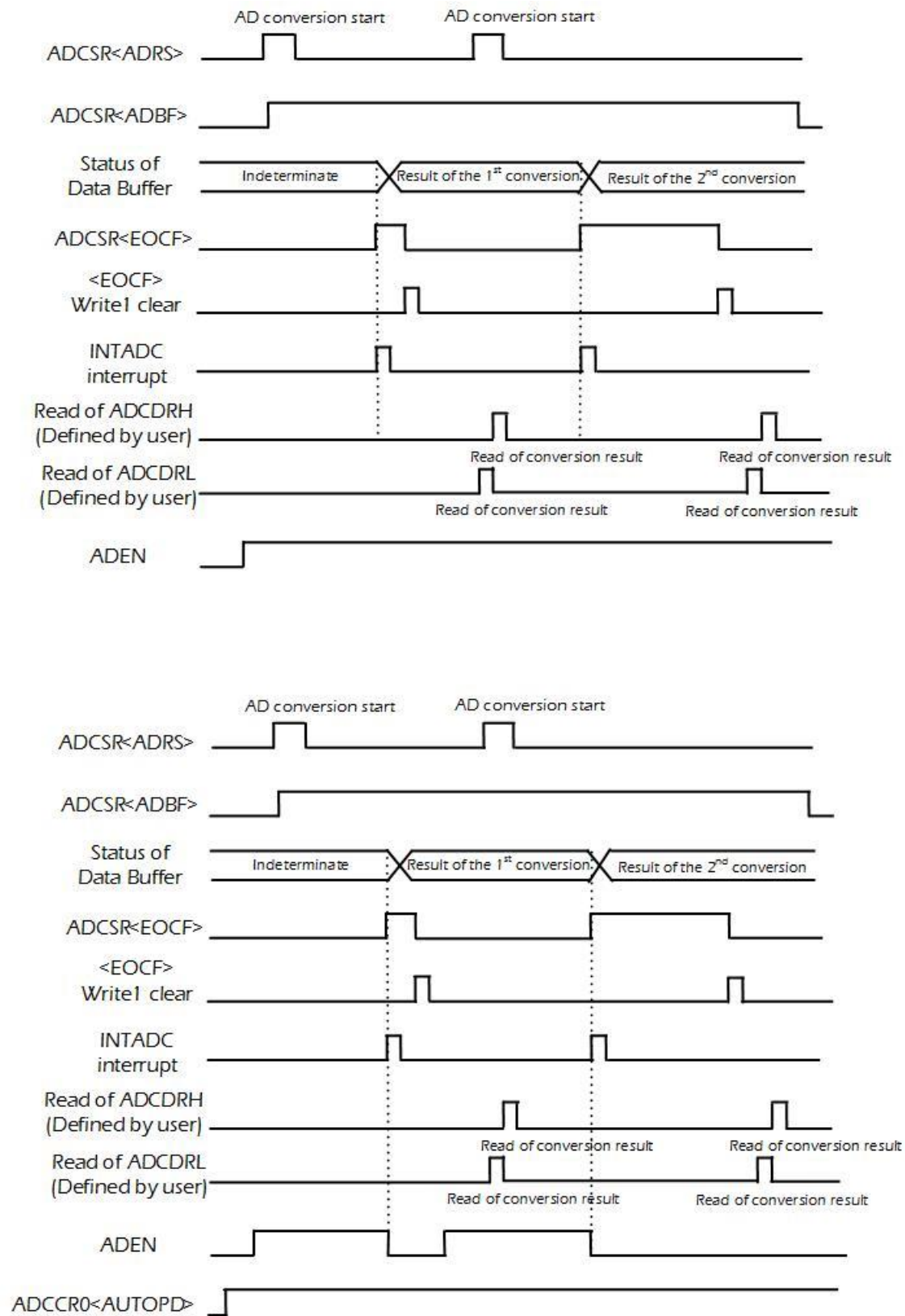
图 8.4 单次模式
