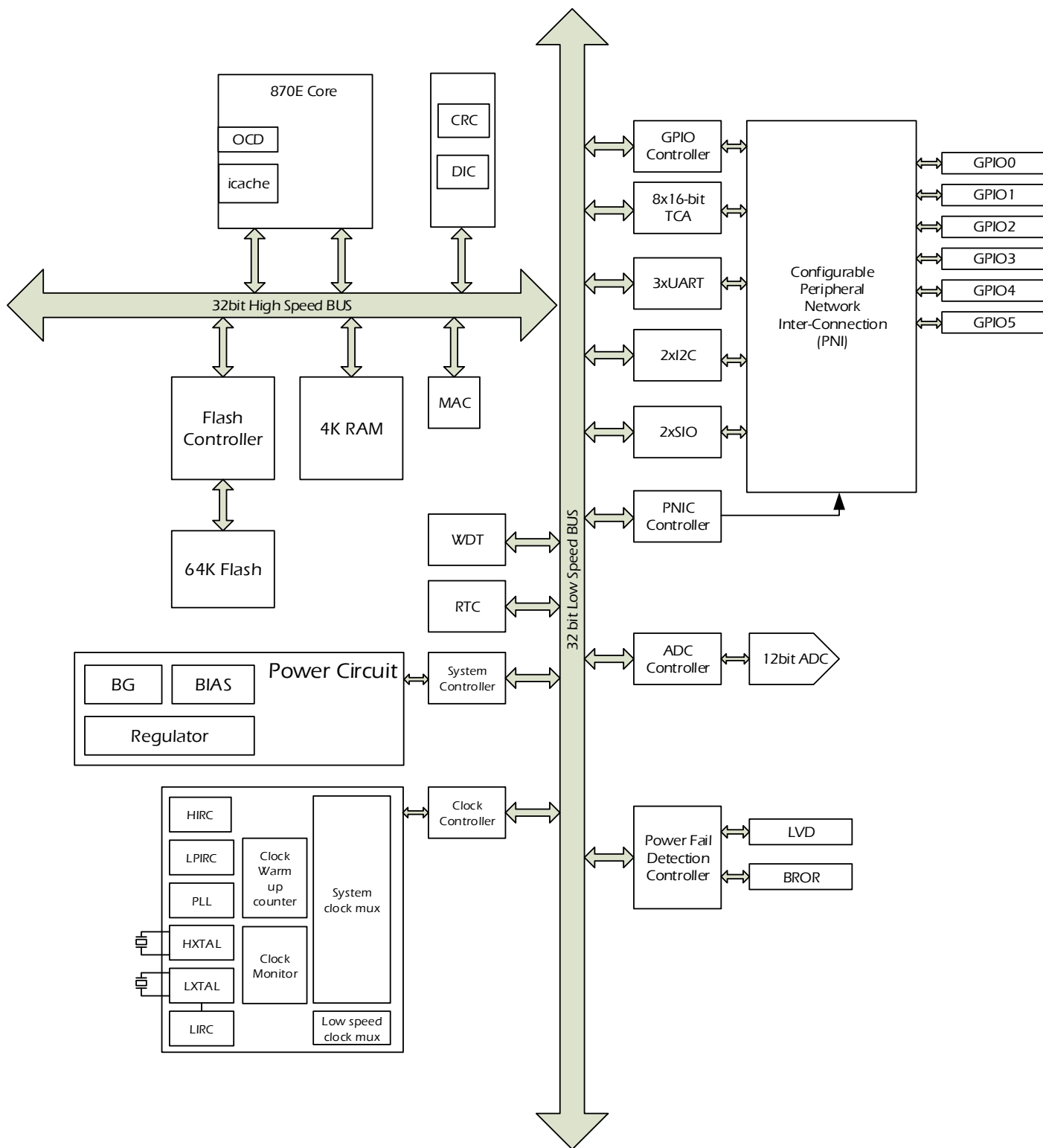
图 2.2 SQ7615系统模块图
