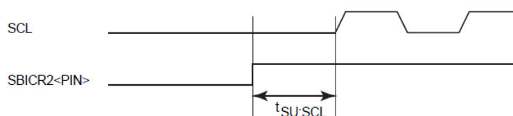
图 15.23 时序定义(No.2)
