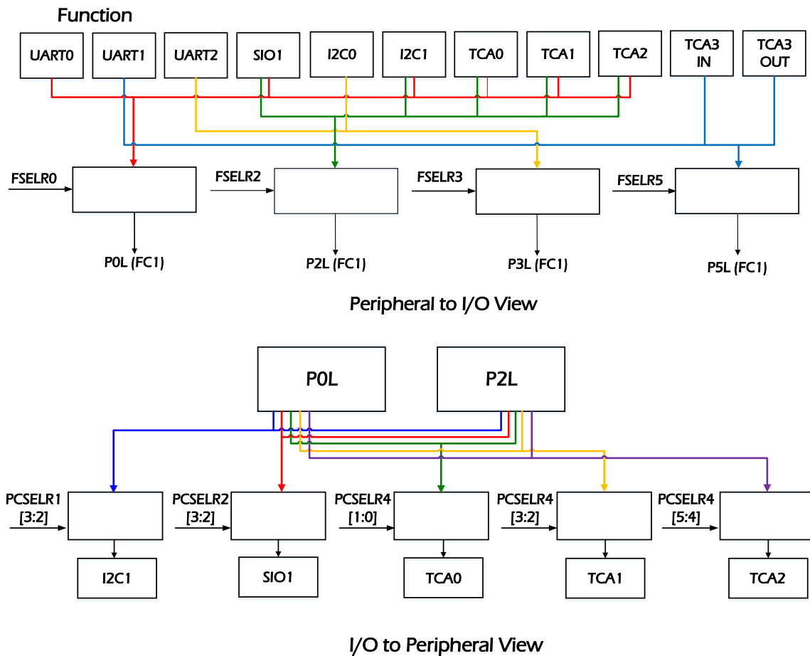
图 12.1 PNIC 架构图
