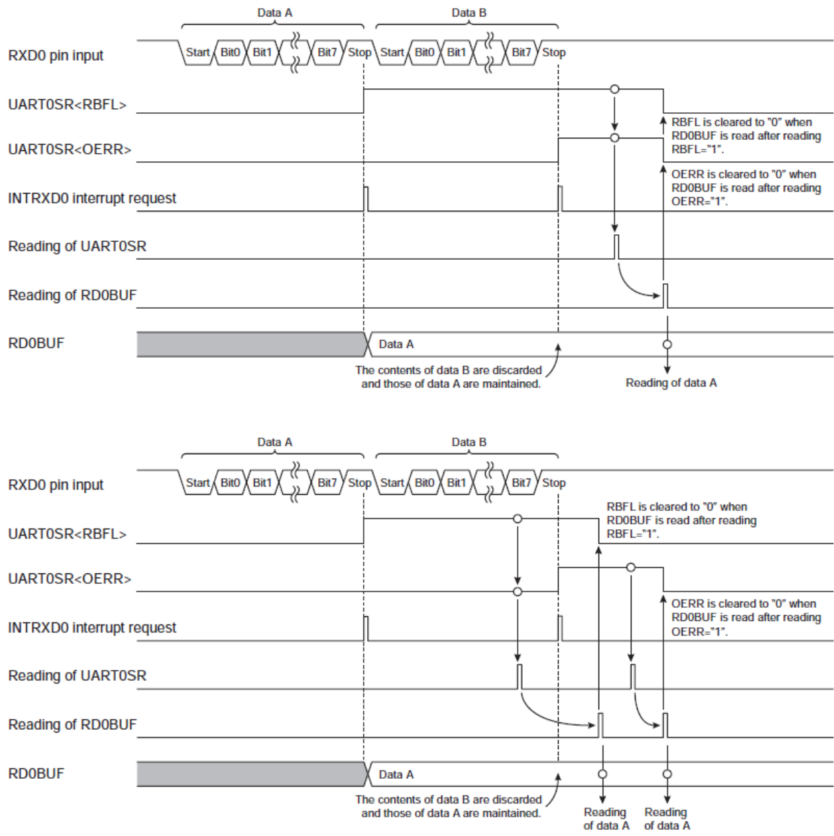
图 14.14 溢出错误标识的清除
