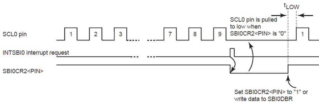
图 15.11 SBIxCR2<PIN>与 SCLx 脚位(以 SBI0 为范例)
