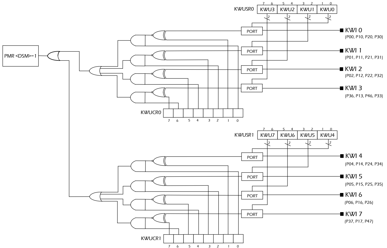
图 6.1 唤醒线路(以 KWI 0~ KWI 7 为例)
