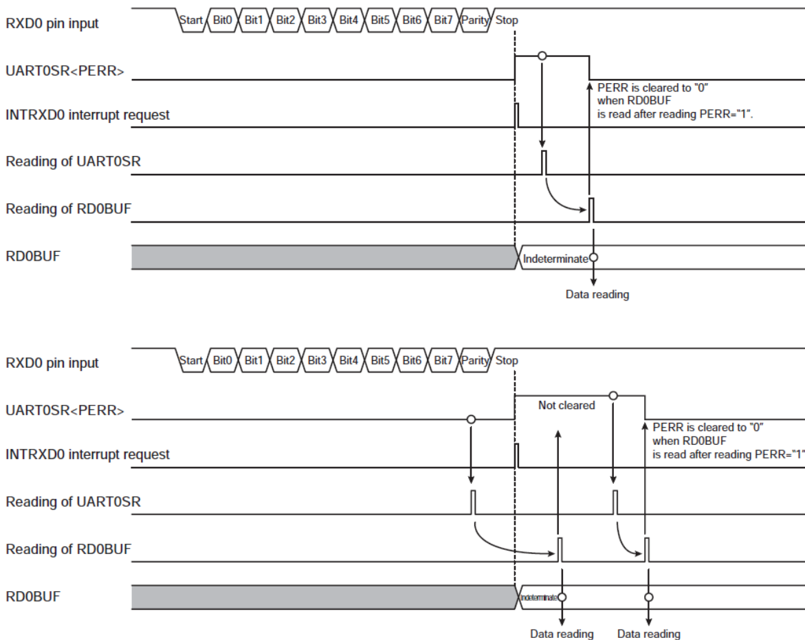
图 14.10 同位错误的发生
