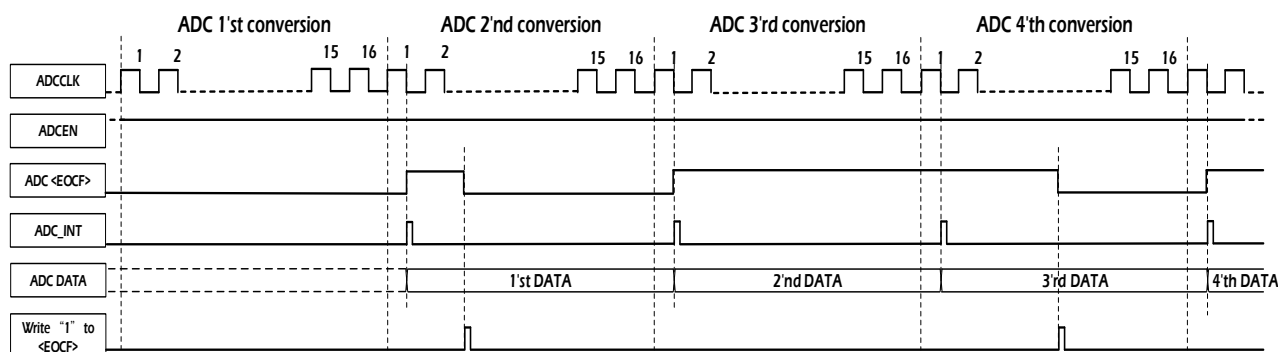
圖 8.3 ADC<EOCF>與數據總線時序圖
