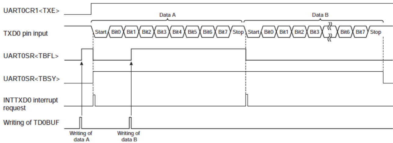
图 14.17 发送缓存器已满的发生
