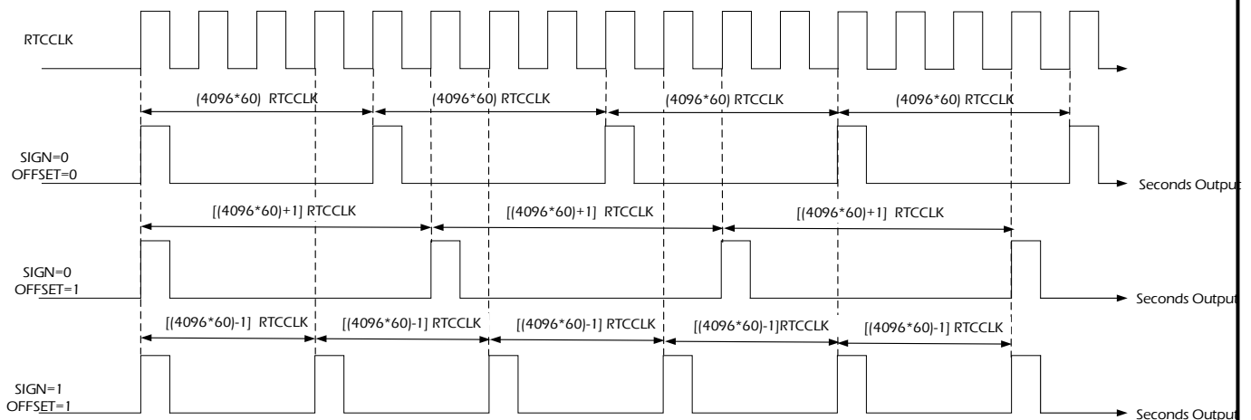
图 13.11 RTC 在 MODE=0 下校正时序范例
