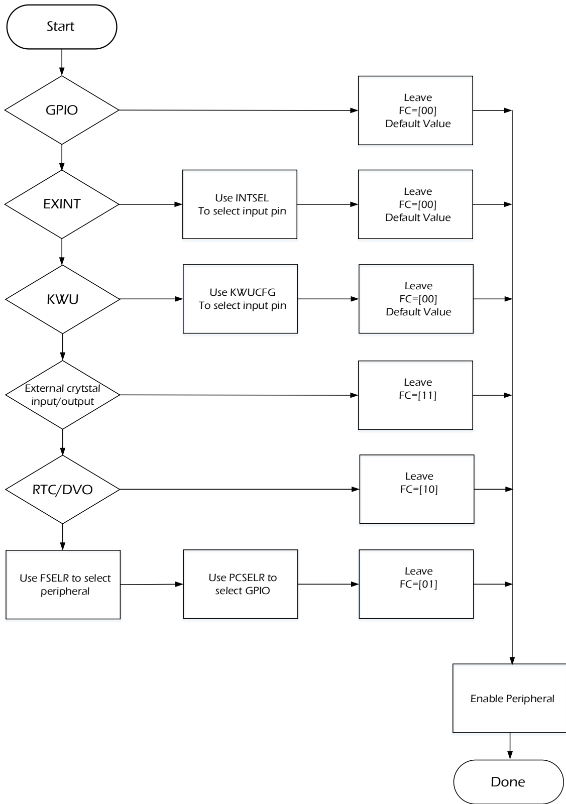
图 12.2 PNIC 操作流程
