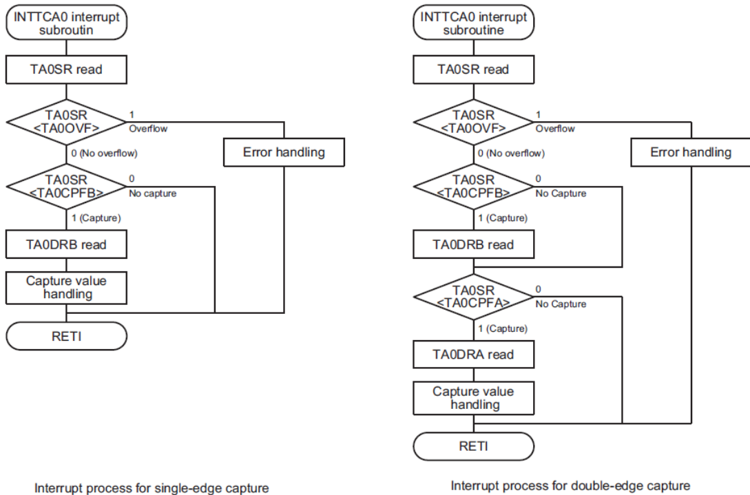
图 13.20 TCA0 抓取进程范例
