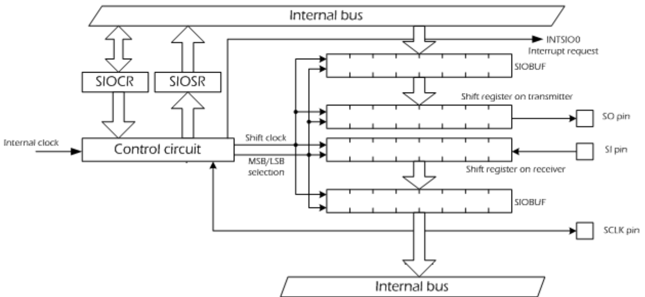
图 16.1 串行接口示意图
