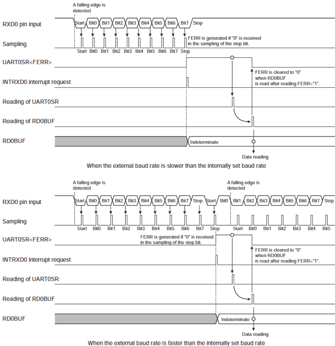
图 14.11 数据框错误的发生
