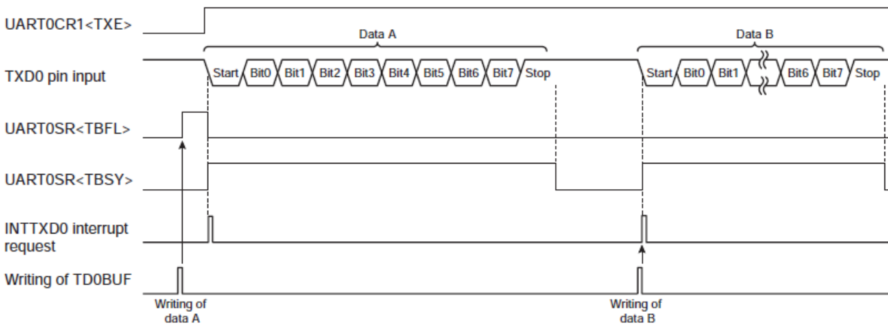
图 14.16 发送数据缓存器已满的发生与发送忙碌标帜
