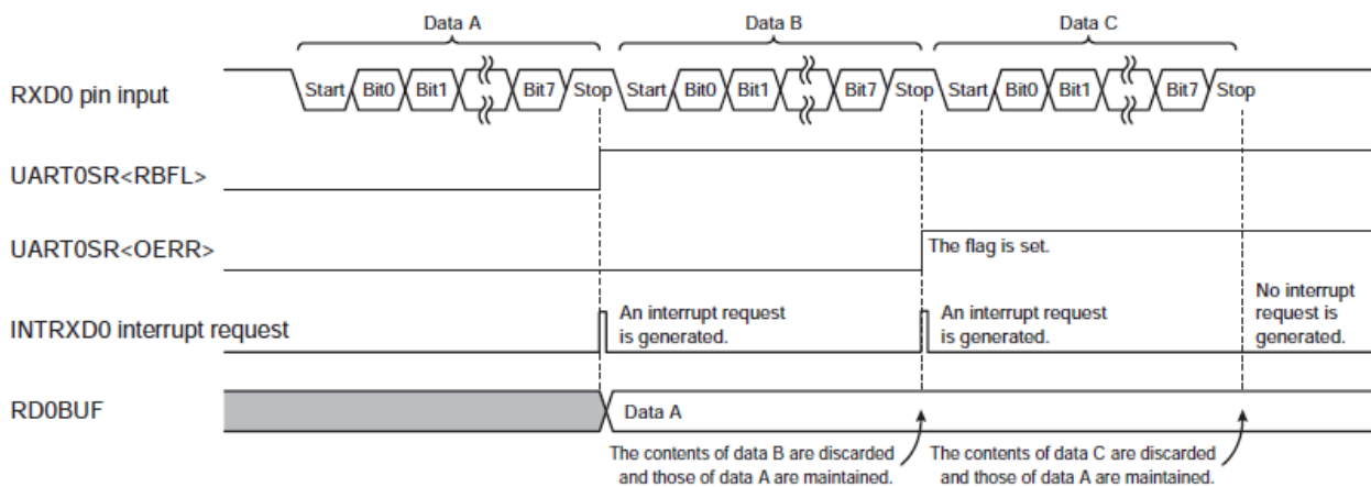
图 14.12 INTRXD0 中断要求的产生
