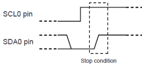
图 15.10 停止条件产生(以 SBI0 为例)
