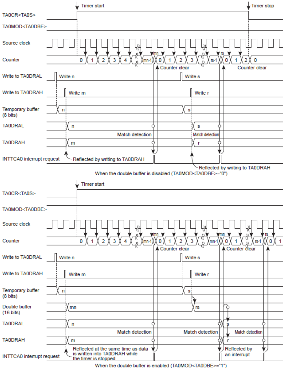
图 13.14 定时器模式时序图(以 TCA0 为范例)
