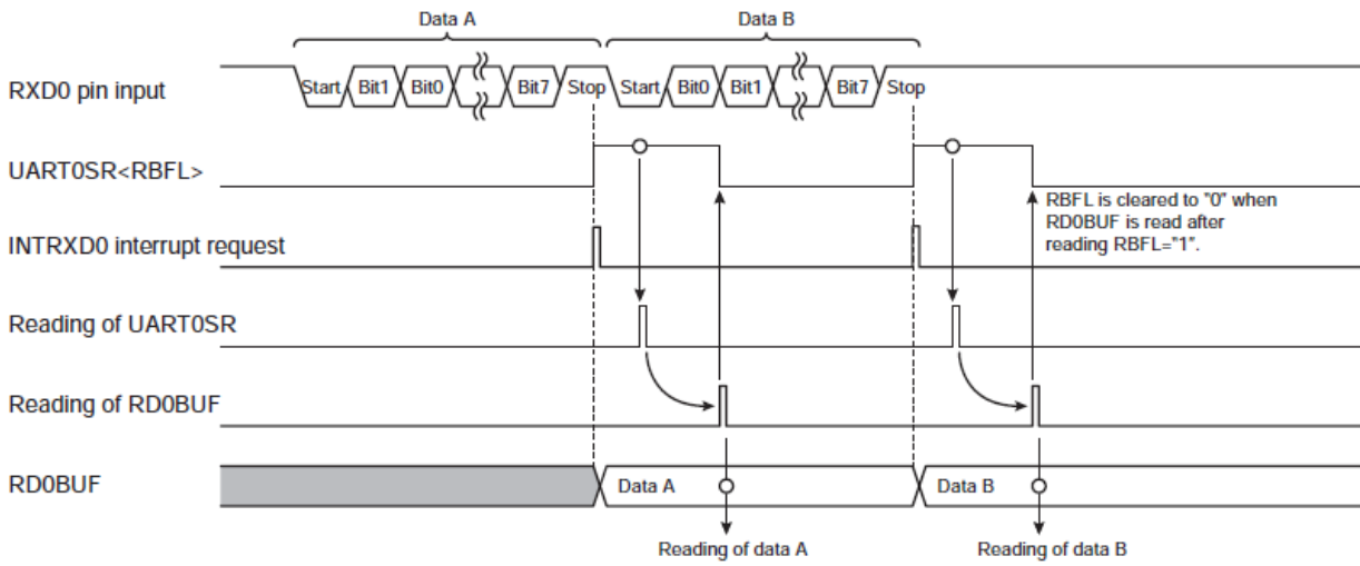
图 14.15 接收缓存器已满的发生
