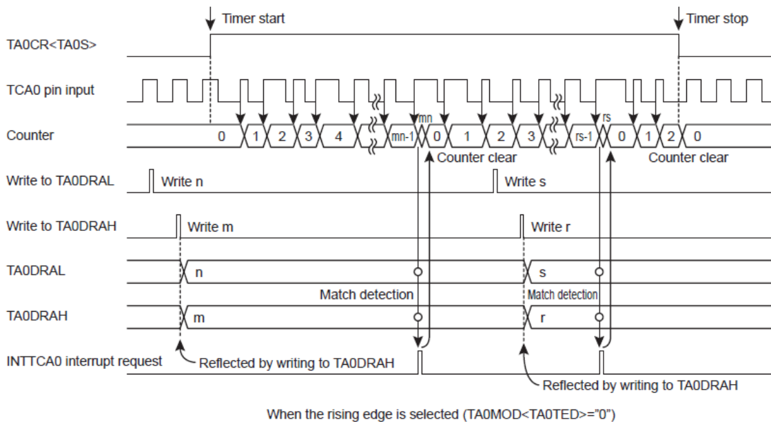
图 13.17 事件计数器模式时序图(TCA0 为范例)
