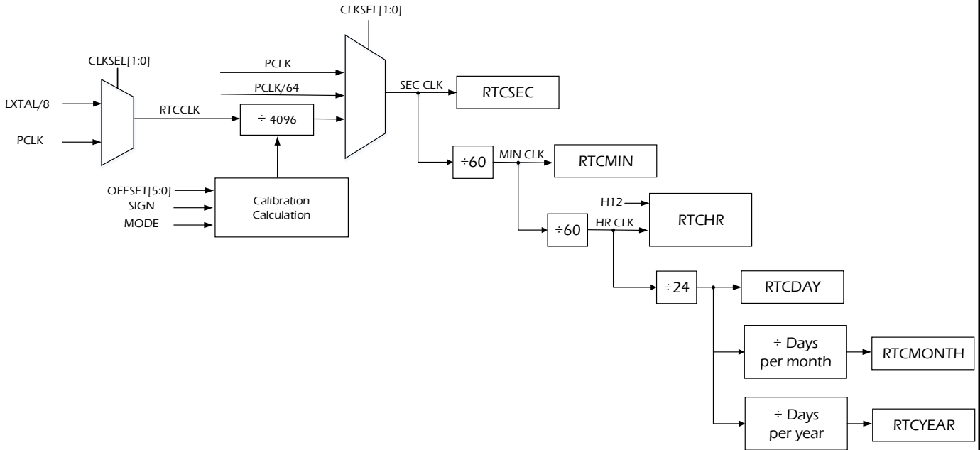
图 13.9 RTC 模块图
