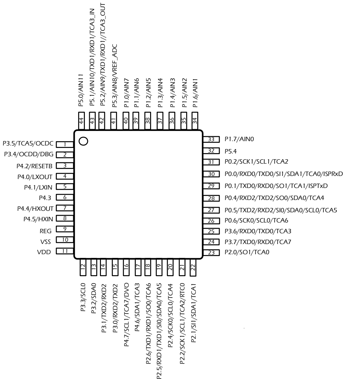
图 2.3 LQFP-44 封装型态引脚配置
