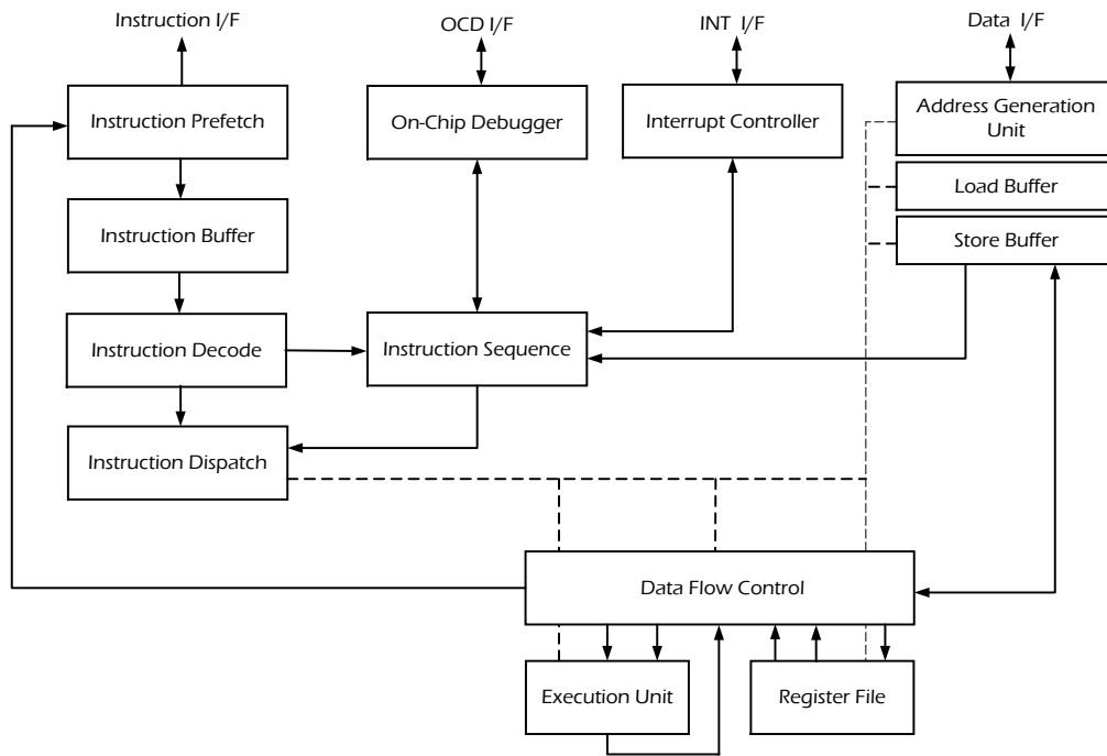
图 2.1 SQ7615 核心工作模块图
