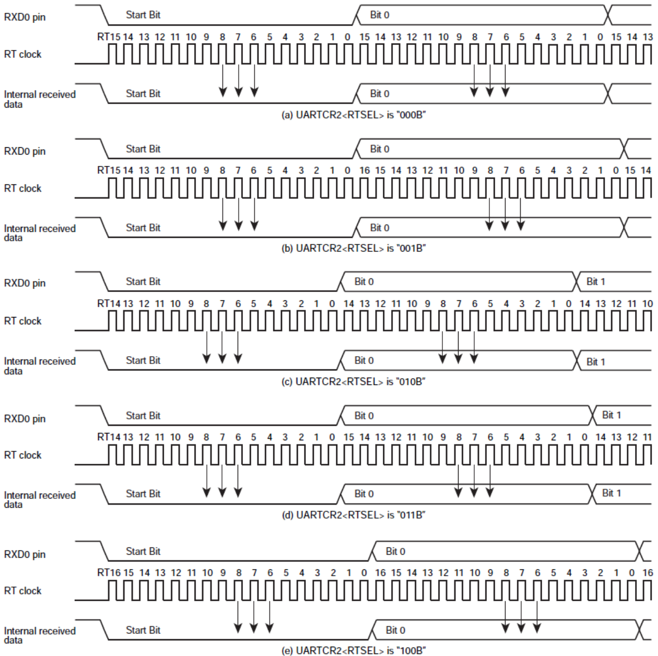
图 14.7 各种 UART0CR2<RTSEL>设定下的数据取样
