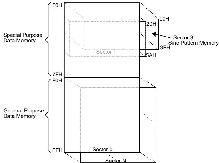
数据存储结构
