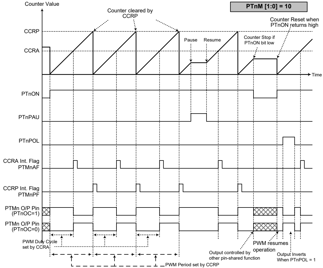
PWM 输出模式 (n=0, 1, 2)
