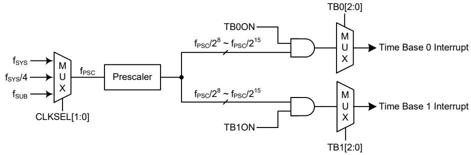
时基中断
