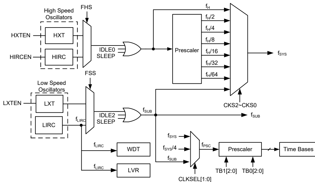
单片机时钟配置
