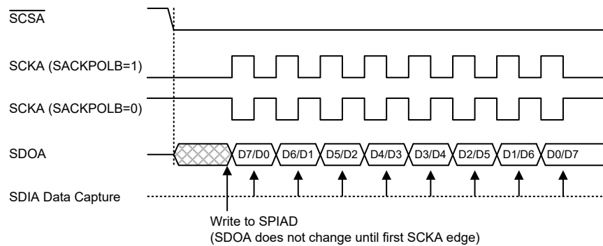
SPIA 从机模式时序图 - SACKEG=0
