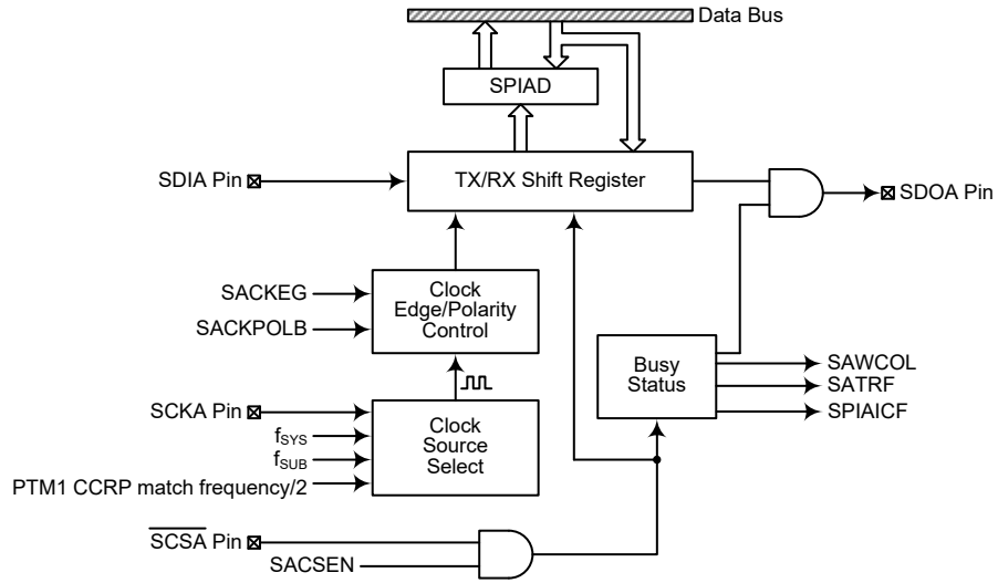
SPIA 方框图
