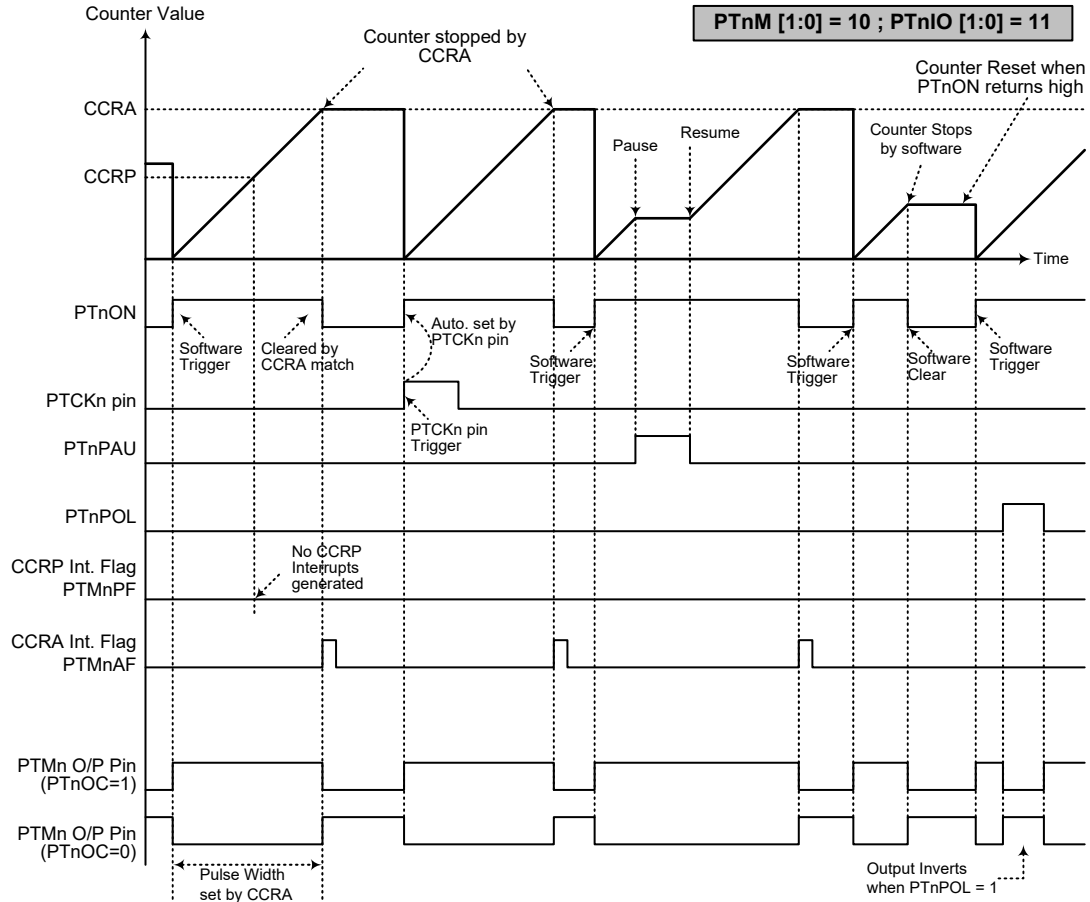
单脉冲输出模式 (n=0, 1, 2)
