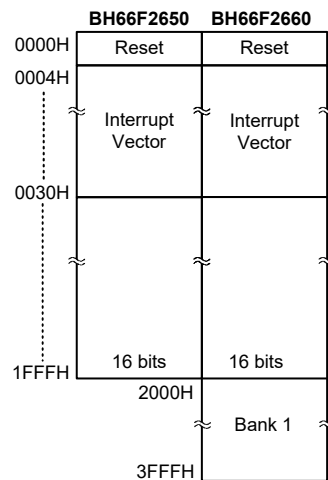
程序存储器结构
