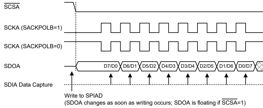
SPIA 从机模式时序图 - SACKEG=1
