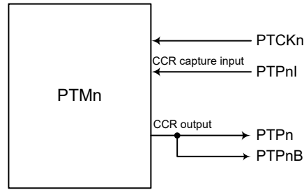
PTM 功能引脚控制方框图 (n=0)
