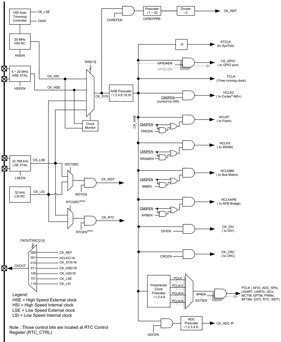
图 3. 时钟结构图
